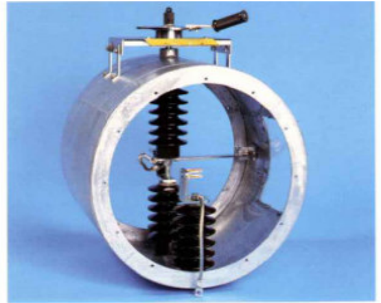
Рисунок 2: GSW 2, разъединительный тип
